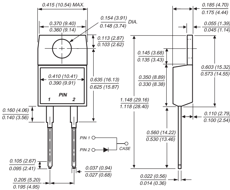
TO-220AC (BYS459)
