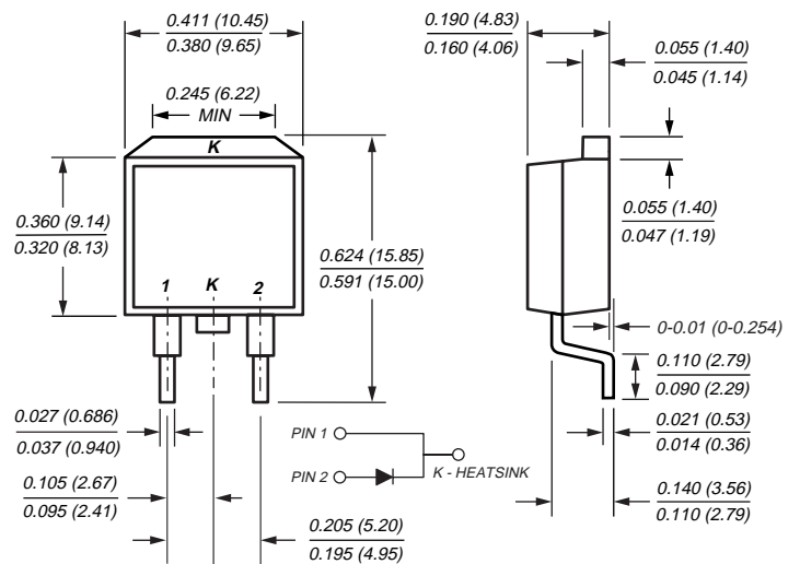
TO-263AB (BYS459B)
